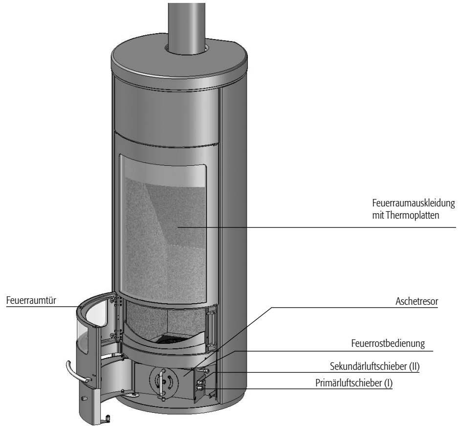
Abb. 1 Bedienungselemente
