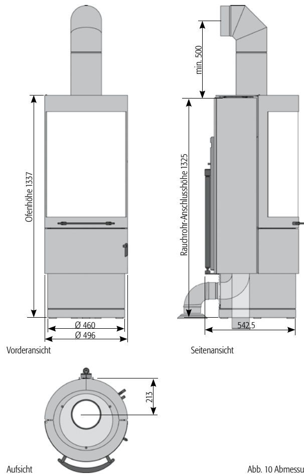
Abb. 10 Abmessungen in mm
