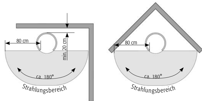
Abb. 3 Grundriss Wandsituation
