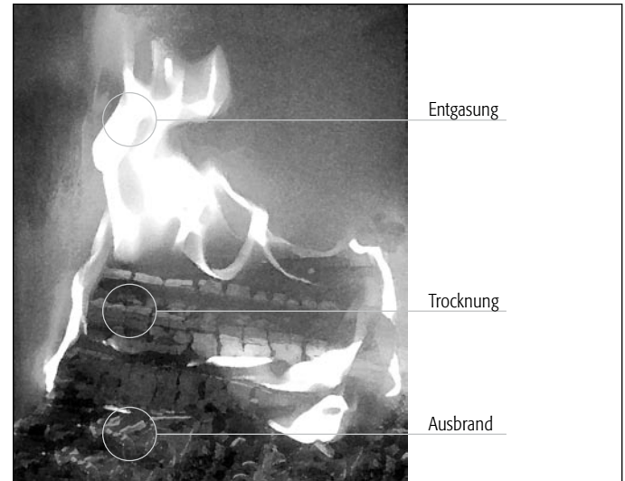
Abb. 7 Der Verbrennungsluftvorgang
