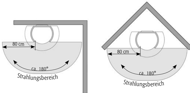
Abb. 5 Grundriss Wandsituation
