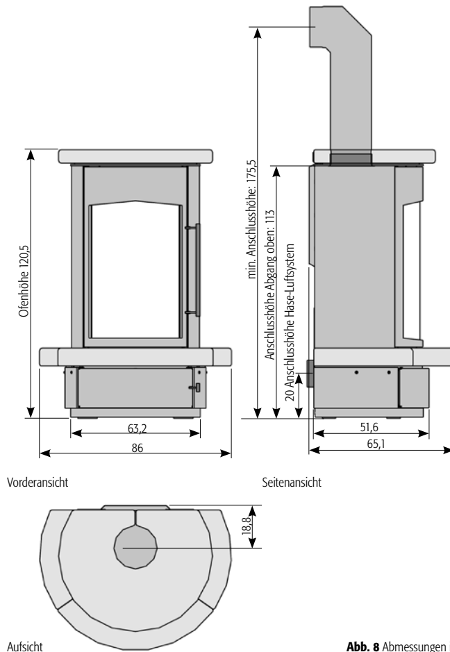
Abb. 8 Abmessungen in cm
