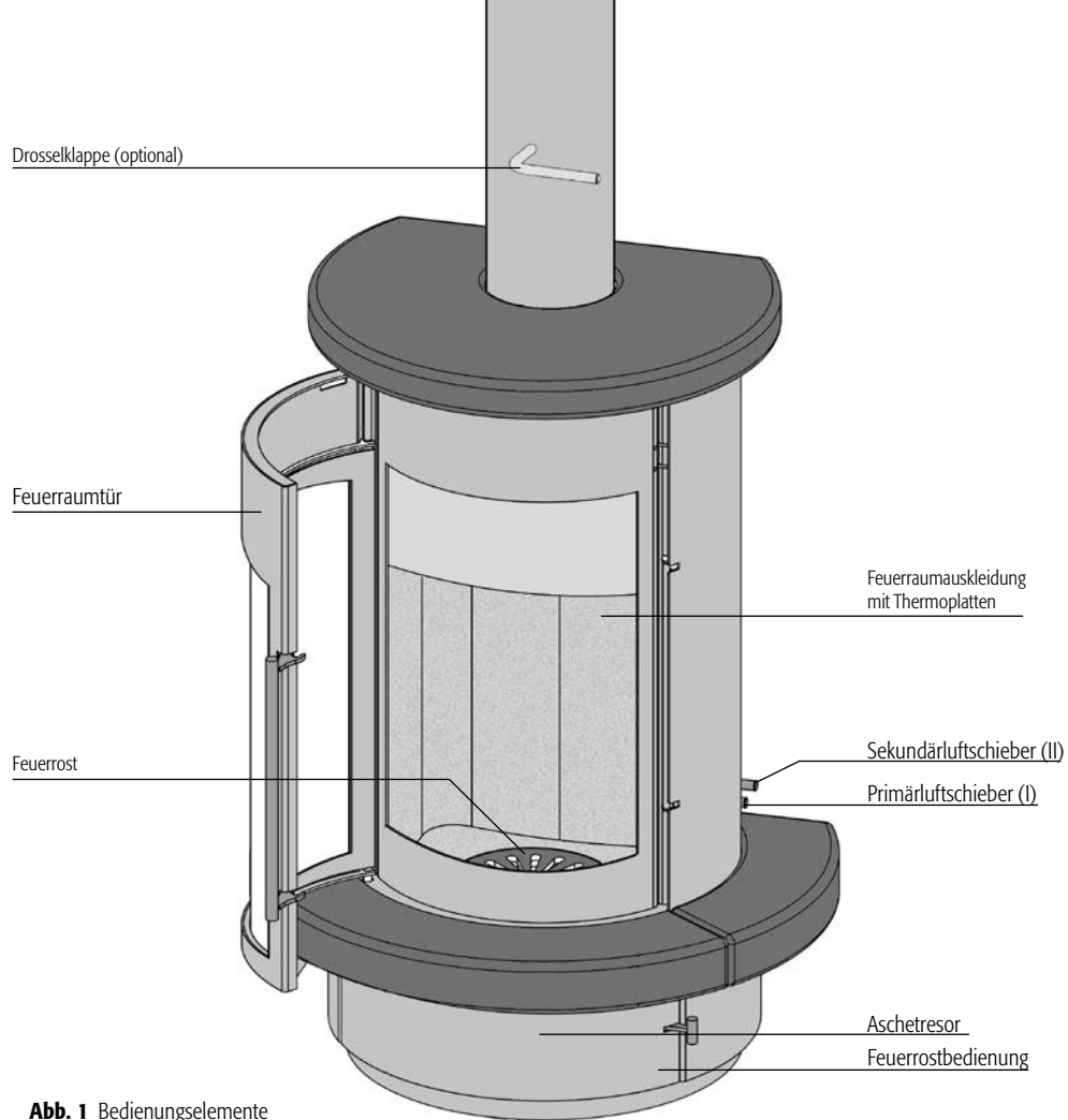
Abb. 1 Bedienungselemente
