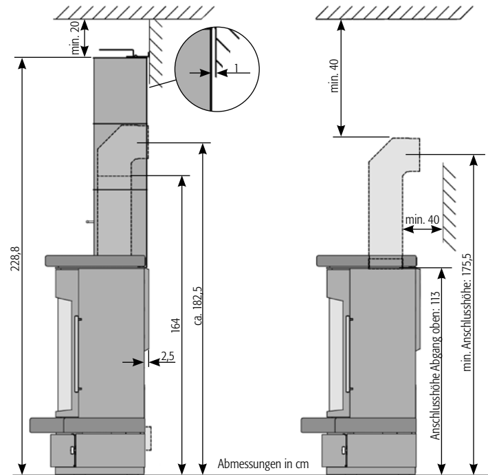
Abb. 2 Aufstellung mit Esse
