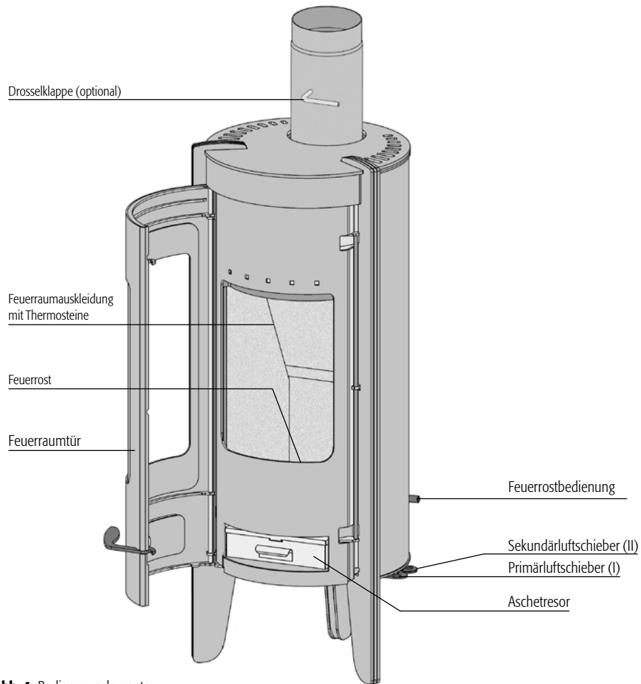
Abb. 1 Bedienelemente
