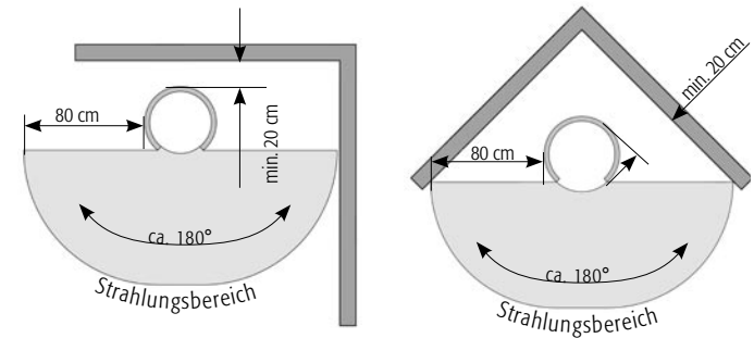
Abb. 3 Grundriss Wandsituation
