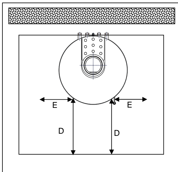
Abbildung Funkenschutzvorlage
