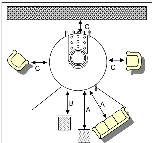
Abbildung Brandschutzabstände
